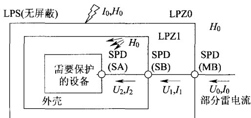
(d)仅采用协调配合好的电涌保护器保护 注：设备得到防线路导入电涌的保护， U_e 大大小于 U_0 和 I_2 大大小于 I_0 ，但不需防 H_0 辐射磁场的保护。
