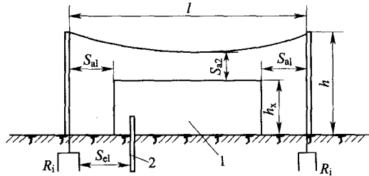
图 4.2.1 防雷装置至被保护物的间隔距离
