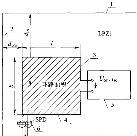
图 G.0.1 环路中的感应电压和电流
