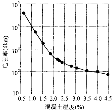
图 12 混凝土湿度对其电阻率的影响
