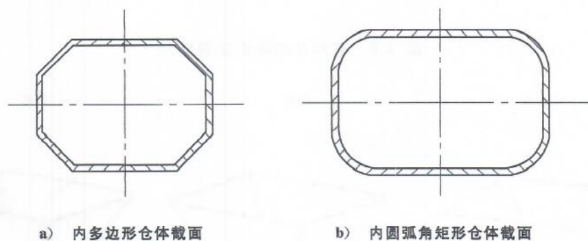
图 A.6 配合饲料粉料仓与成品仓体截面
