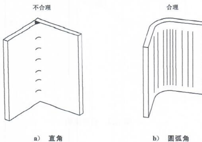
图 A.7 粉料仓和成品仓体的棱角处理
