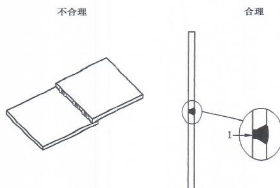
图 A.10 仓斗拼接焊缝
